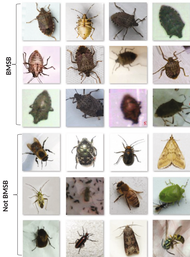
Fig. 5. Dataset samples.
