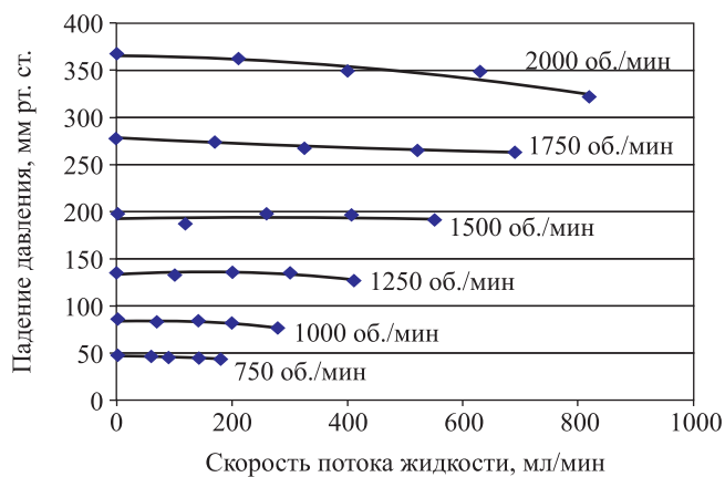
Рис. 6. Падение давления в зависимости от скорости потока жидкости (водный раствор карбоксиметилцеллюлозы вязкостью 3,3–3,5 сантипуаз) при различных значениях скорости кровотока в устройстве Nemolung
